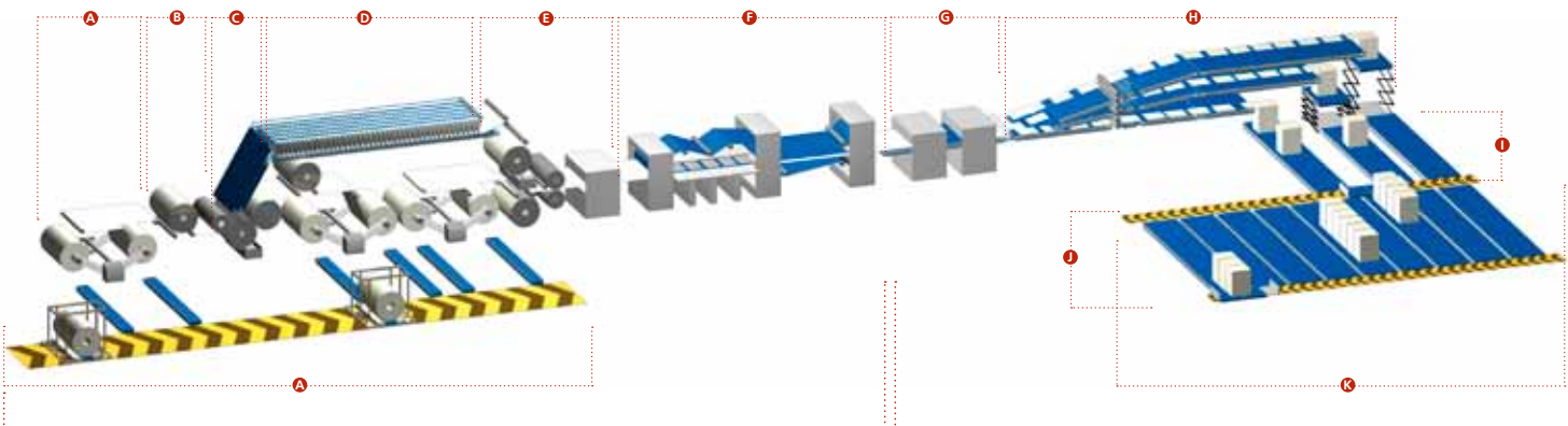
Wellpappenanlage
